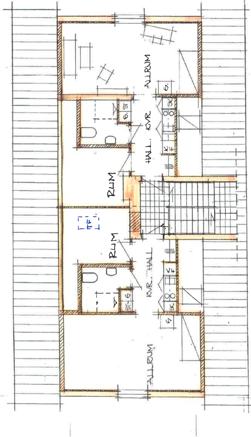
VINDSPLAN
